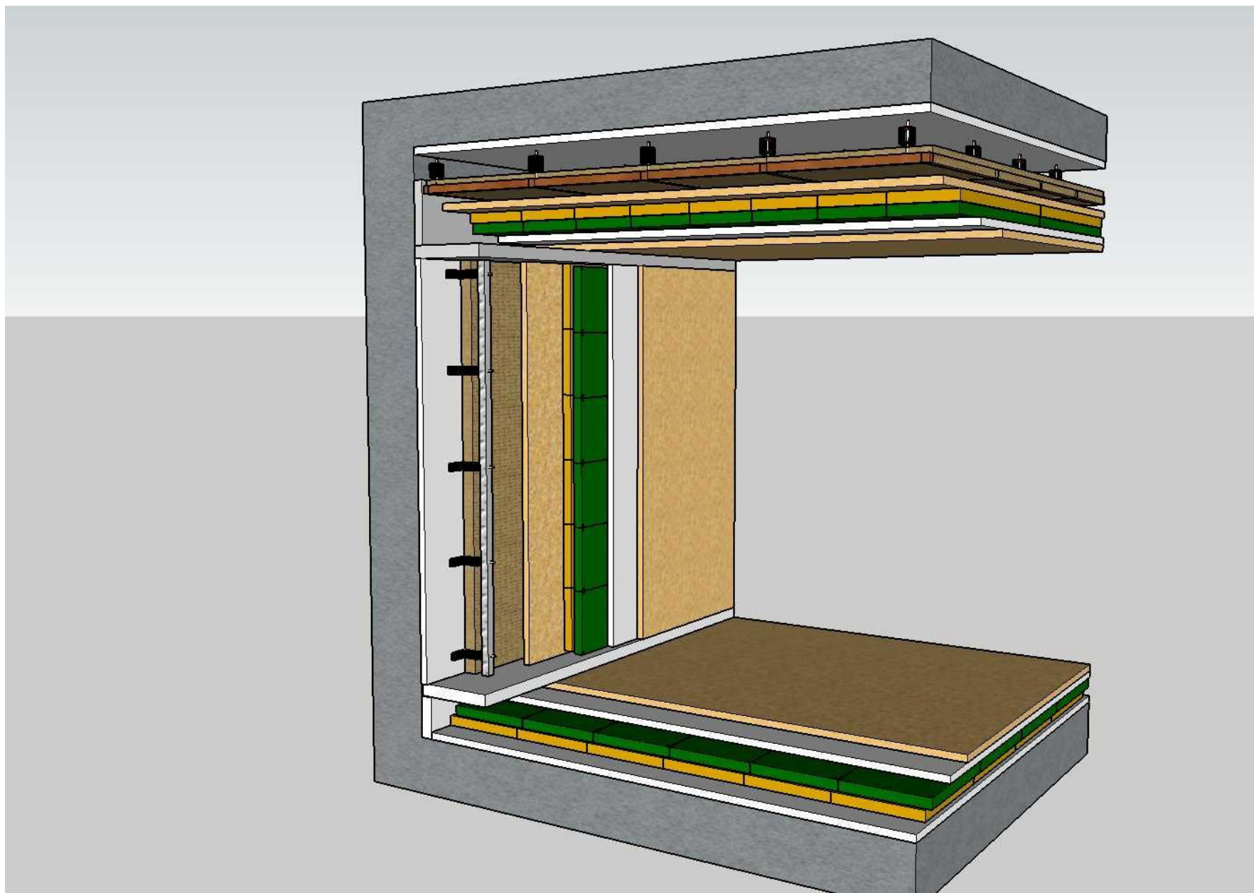
总体隔音减震结构示意图
