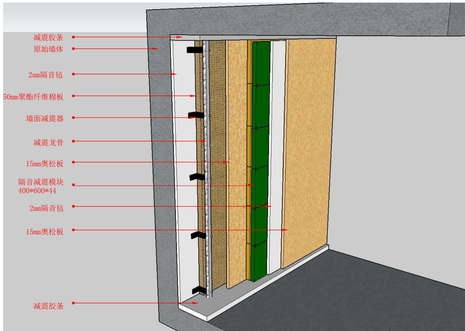
墙面隔音减震结构示意图
