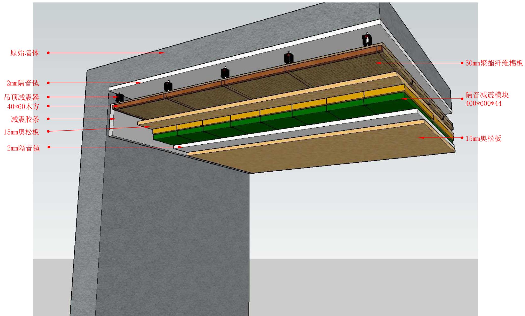
顶面隔音减震结构示意图
