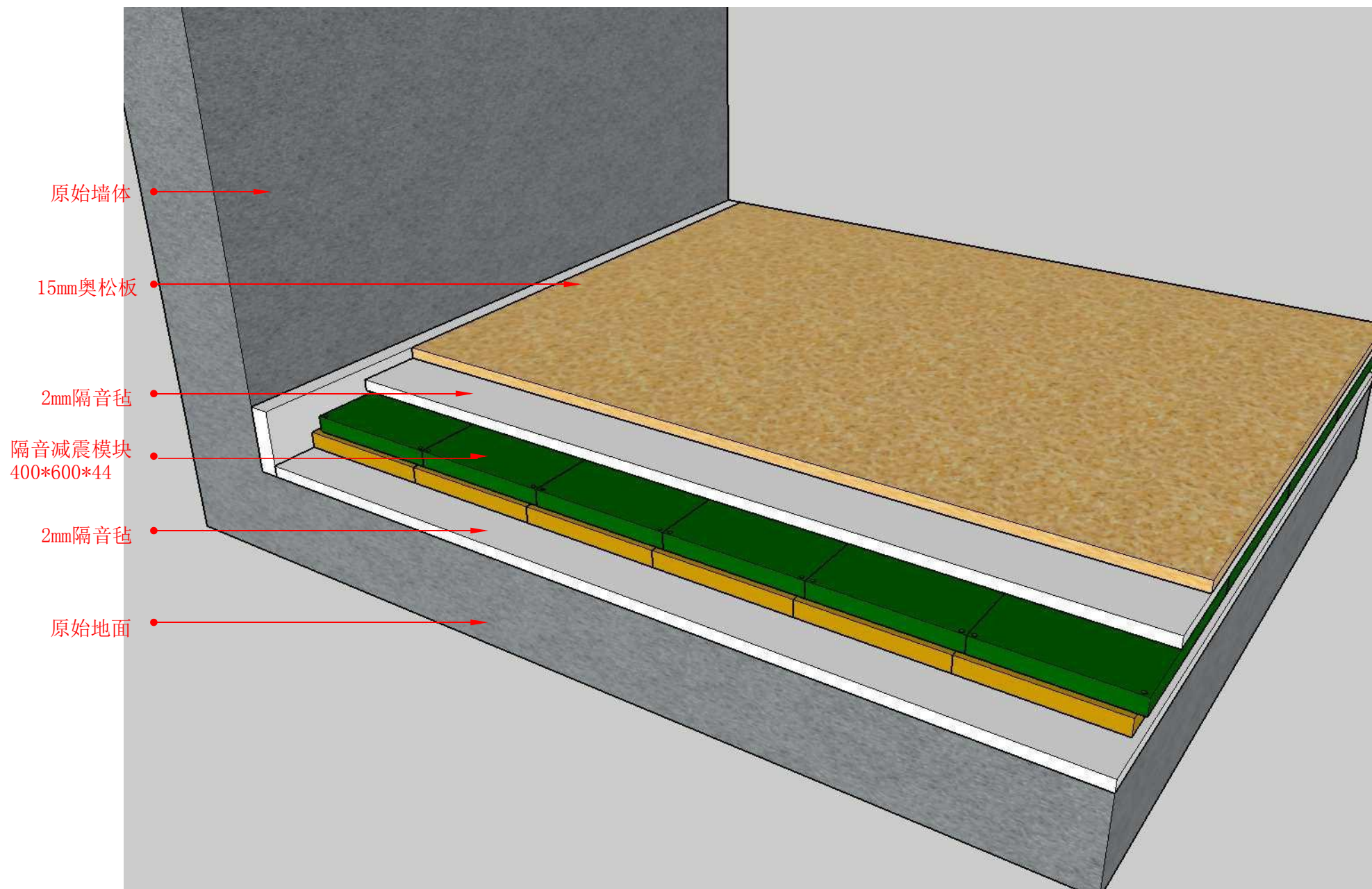
地面隔音减震结构示意图
