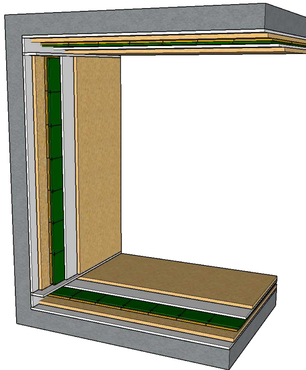
整体隔音结构示意图
