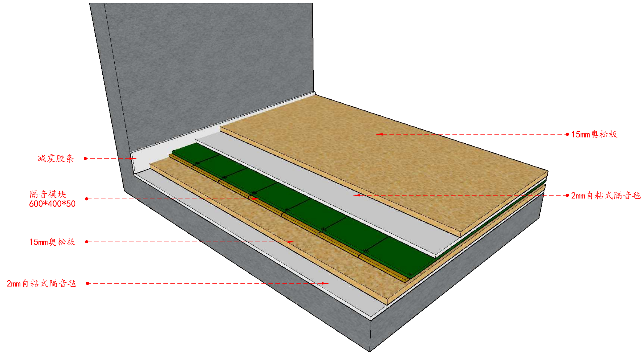
地面隔音结构示意图
